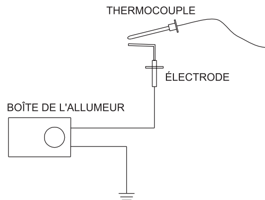
Figure 37 – Câblage du système allumeur électronique
