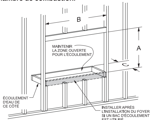
DIMENSIONS DE L'INSERTION (en pouces)
