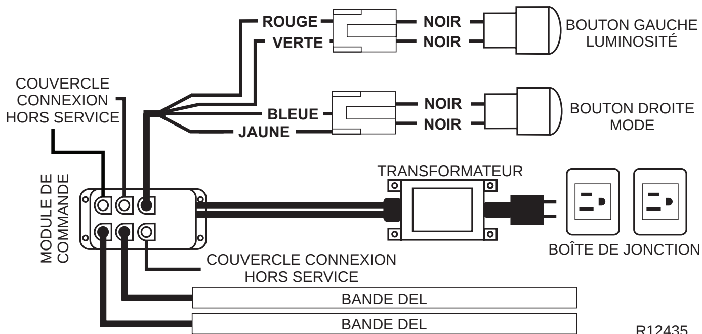
Figure 36 – Câblage du système DEL
